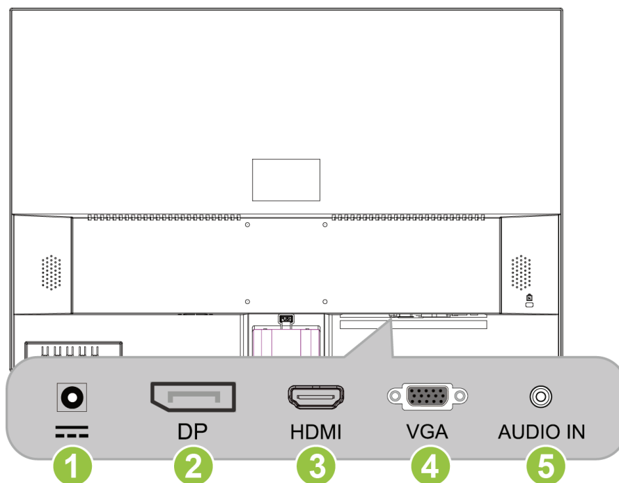
Figura 2. Branchement à un pc
